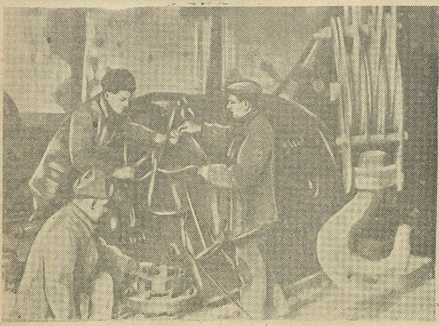
На гомельскай электрастанцыі. На здымку: слесары-монтажнікі за зборкай новага турбагенератара. Фото А. Карніцкага.
